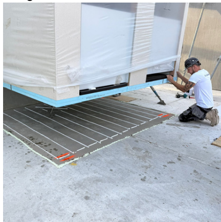
20. Prefab badkamer wordt geplaatst.
